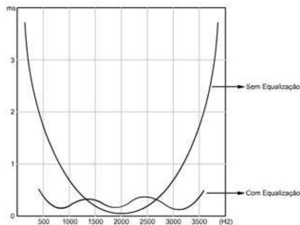
Figura 2.9 – Sinal com e sem equalização
