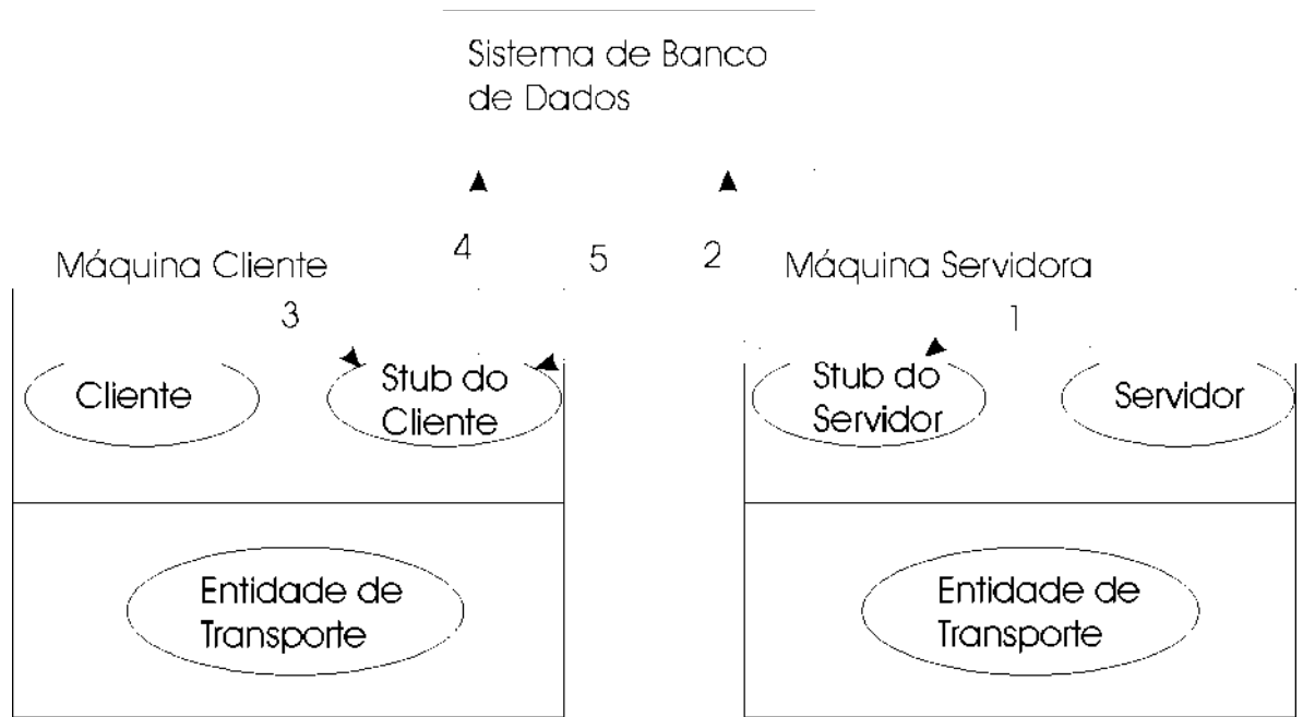
Figura 14-15 A vinculação cliente-servidor é feita através de um banco de dados
