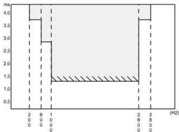
2.8 - Variação permissível do retardo
