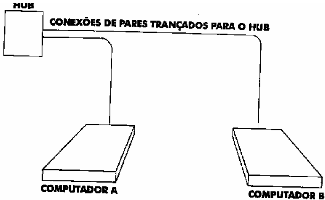
Figura 2.6 Ilustração de uma fiação de pares trançados utilizada pela Ethernet. Cada computador conecta-se a um HUB por cima de um par de fios
