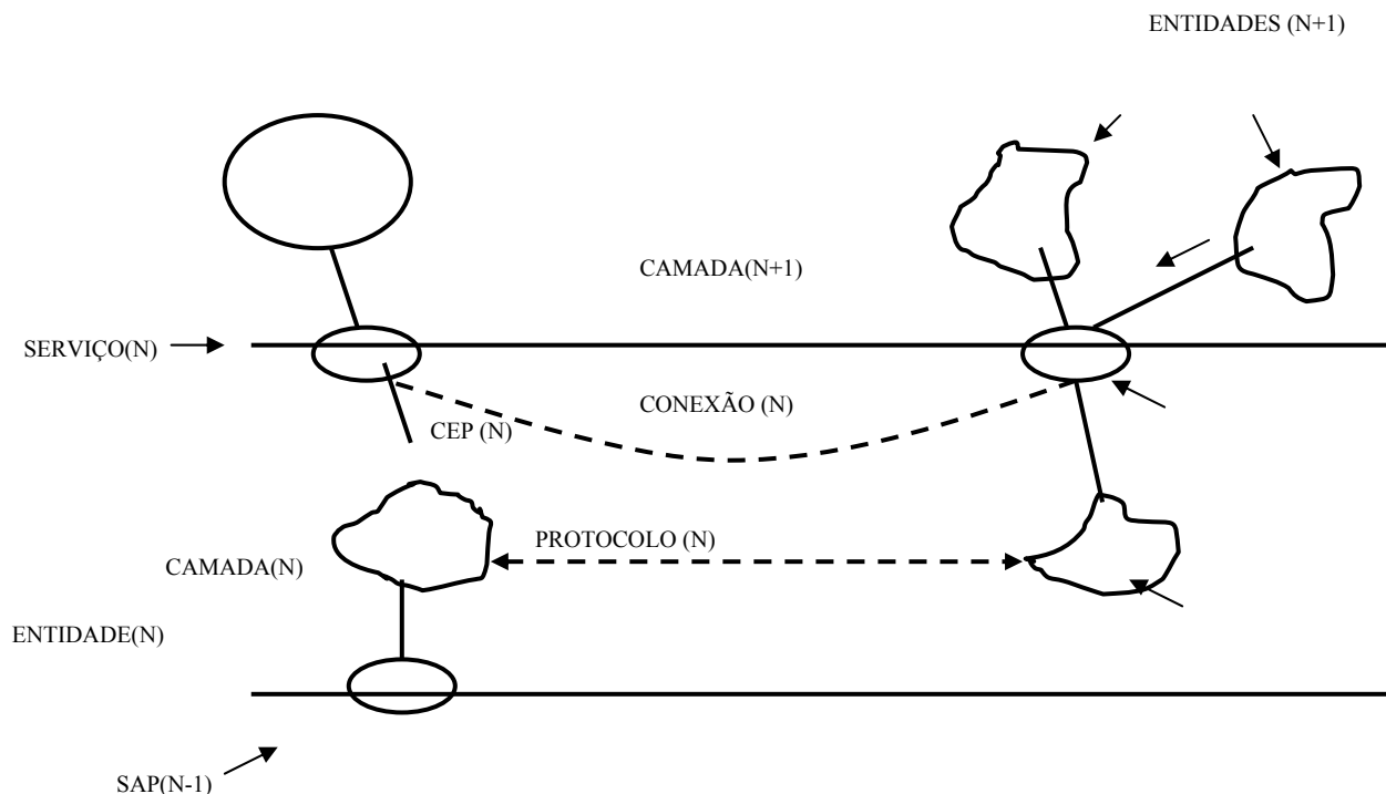
Figura 7.4: Ilustração de alguns termos do RM-OSI da ISO.
