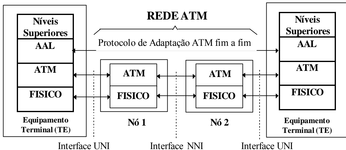
Figura X.3. Modelagem de uma rede ATM segundo o modelo PRM da I.321.
