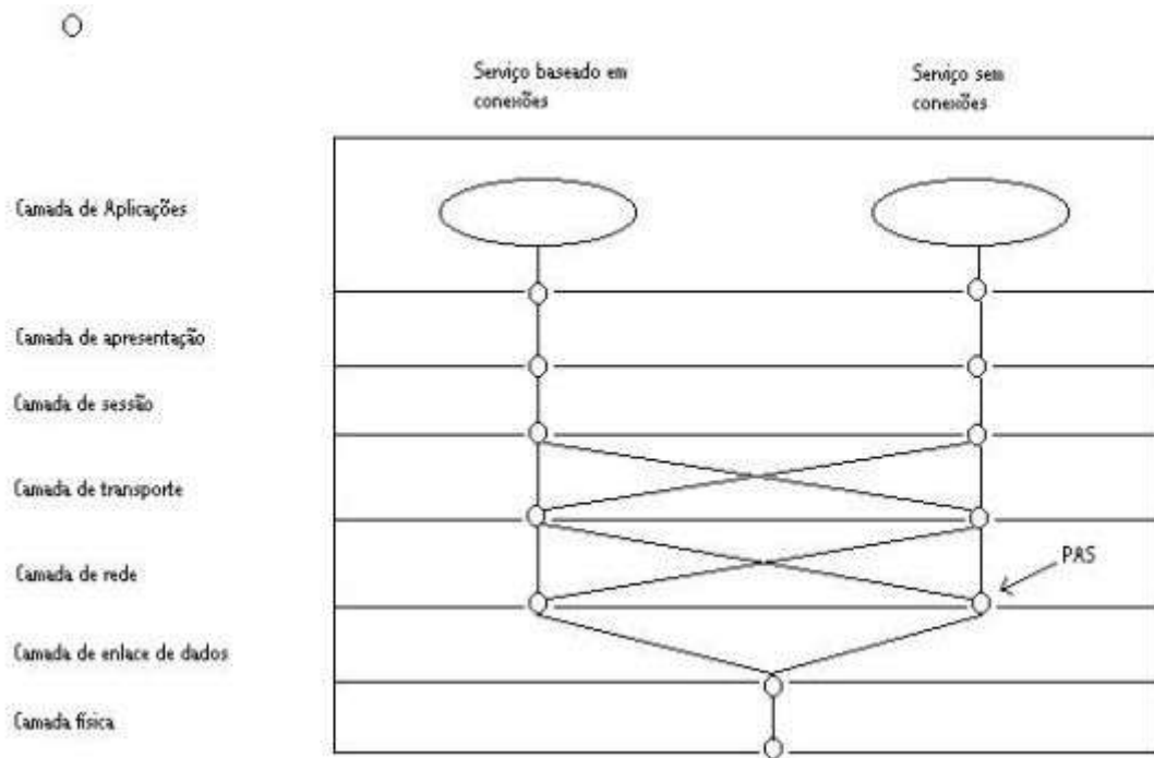
Figura 10-2 Misturas de serviços baseados em conexões e serviços sem conexões no modelo OSI
