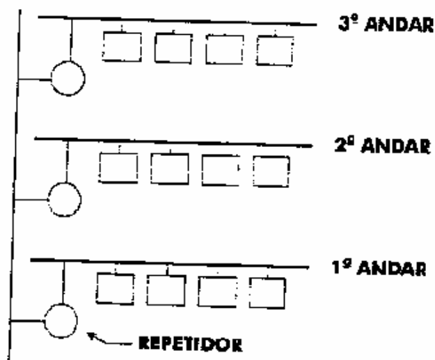
Fig 2.9 Repetidores utilizados para unir os cabos da Ethernet num edifício. No máximo dois repetidores podem ser posicionados entre um par de comunicantes entre si.
