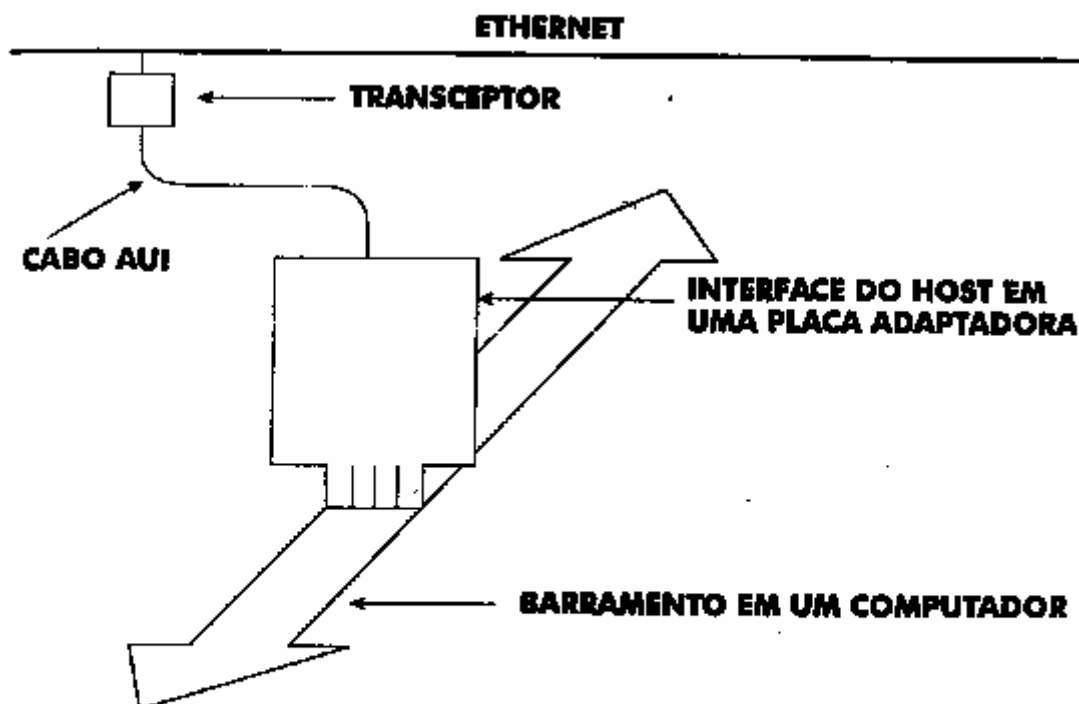
Figura 2.3 Os dois principais componentes eletrônicos que formam uma conexão entre um barramento de computador e uma Ethernet. O cabo AUI que conecta a interface do host ao transceptor transporta a energia elétrica e os sinais para controlar a operação do transceptor, assim como dos pacotes que estão sendo transmitidos ou recebidos
