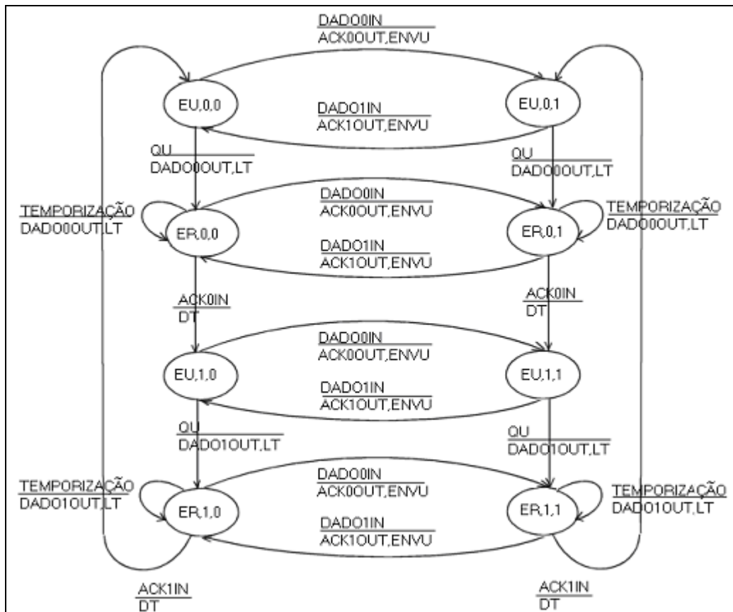
Figura 8.3 – Diagrama de Estados
