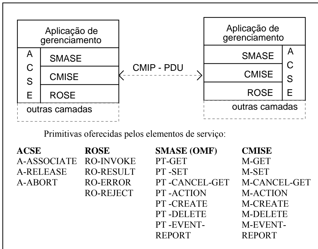
Figura 17.2 - Elementos de Serviço para o suporte às aplicações de gerenciamento
