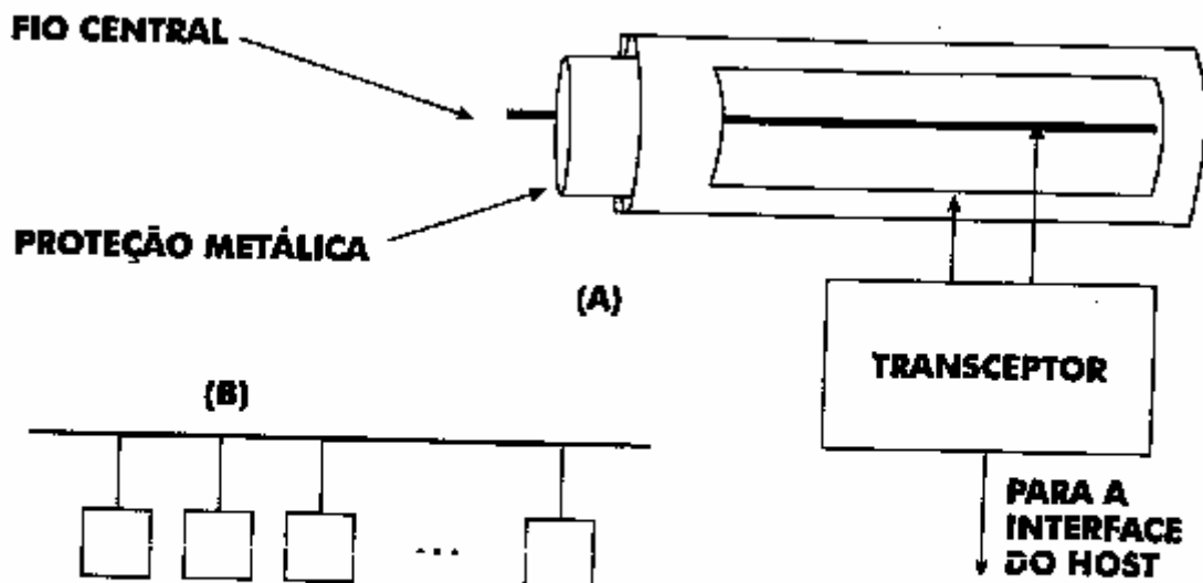
Figura 2.2 (a) Um corte transversal em um cabo Ethernet, mostrando os detalhes dos componentes elétricos entre o transceptor e o cabo, e (b) o diagrama esquemático de uma Ethernet com vários computadores conectados
