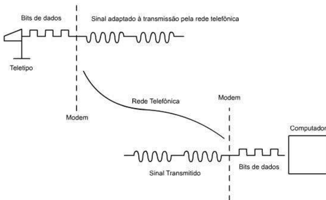
Figura 2.3 - Rede com Modem
