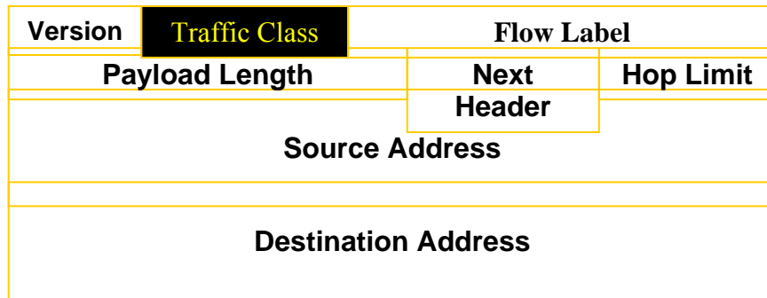
Figura 8: Modelo Cabeçalho do Ipv6 [44]
