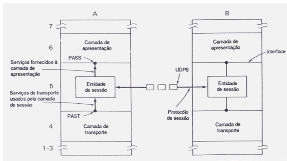
Figura 14.1. As camadas de Transporte, Sessão e Apresentação.
