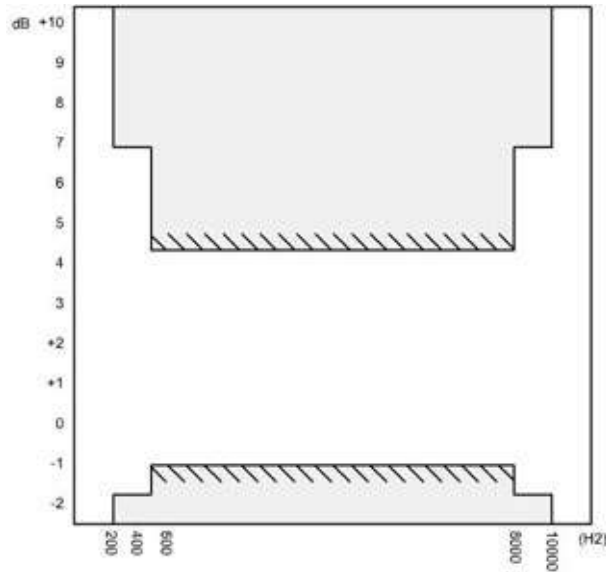
Figura 2.7 - Variação permissível da atenuação
