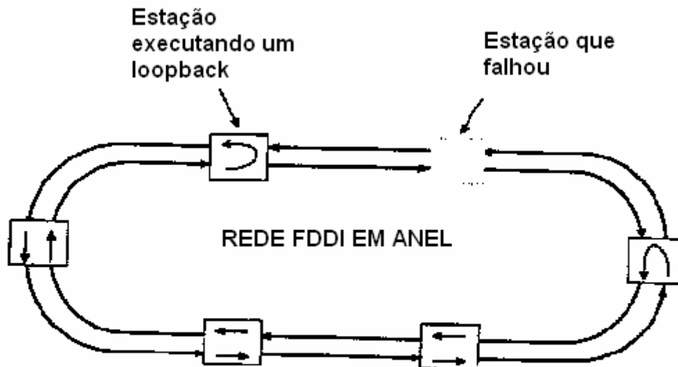
Fig. 2.11 Um anel da FDDI após a ocorrência de uma falha. Quando o hardware da FDDI detecta uma falha, utiliza o segundo anel para contorná-la e permite que as outras estações se comuniquem
