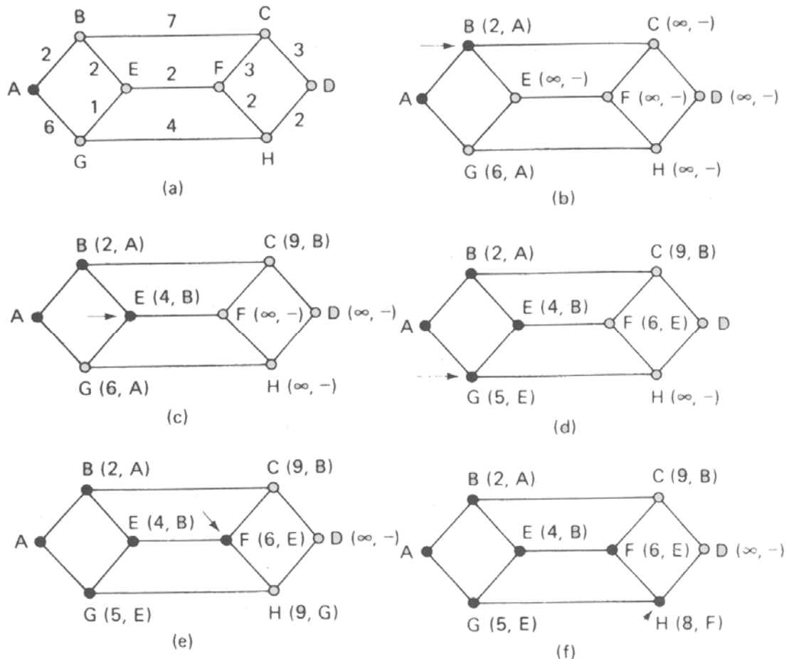
Figura 10.10. As cinco primeiras etapas usadas na computação do caminho mais curto de A para D. As setas indicam o nó de trabalho.
