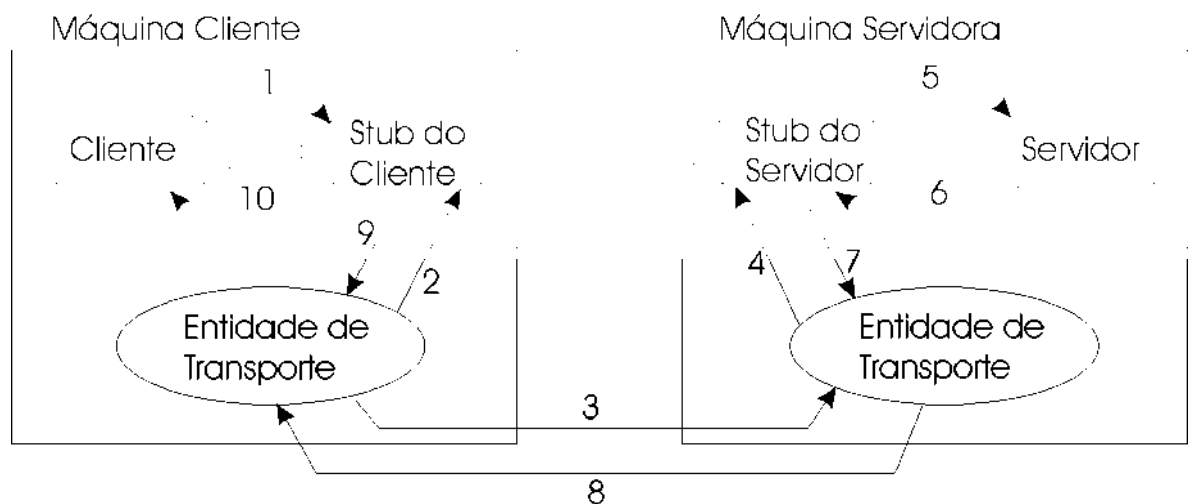
Figura 14-13. As dez etapas necessárias para a execução de uma chamada a procedimento remoto
