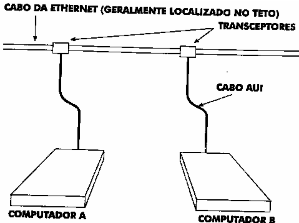
Figura 2.4 A conexão física entre dois computadores a uma Ethernet com o esquema original de fiação. Em um ambiente de trabalho, o cabo da Ethernet é normalmente localizado junto ao teto do corredor; cada sala possui um cabo AUI que conecta um computador do escritório a um transceptor ligado ao cabo da Ethernet
