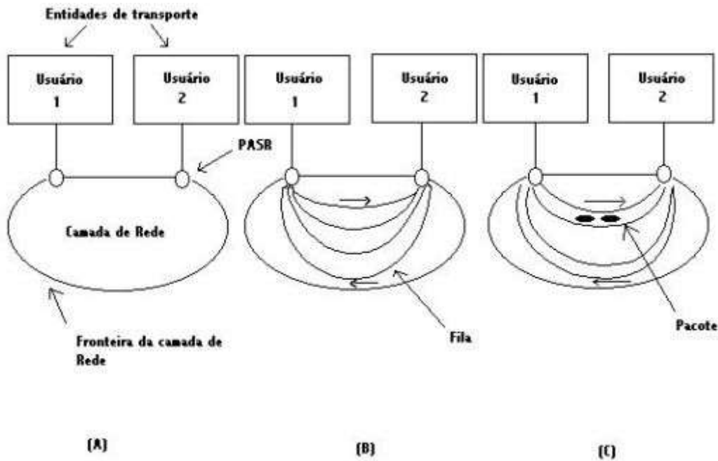
Figura 10-3 (A) Antes de estabelecer uma conexão (B) Depois de estabelecer uma conexão (C) Depois que dois pacotes são enviados, mas ainda não recebidos.
