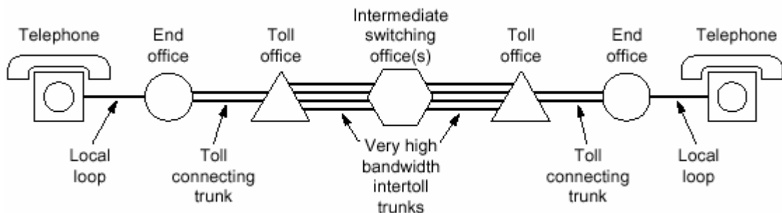
Figura 19.3 - Rota de um circuito típico de uma chamada a média distância.
