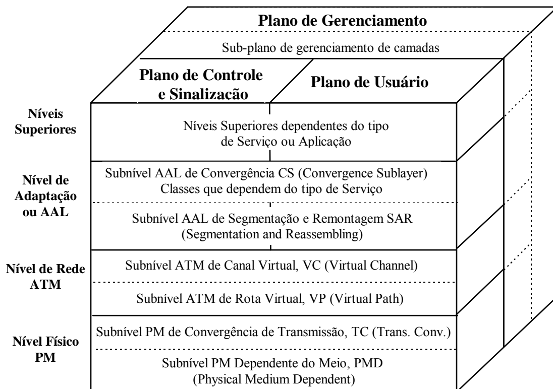
Figura 2.2 - Modelo de Referência de Protocolos da B-ISDN segundo a Rec. I.321
