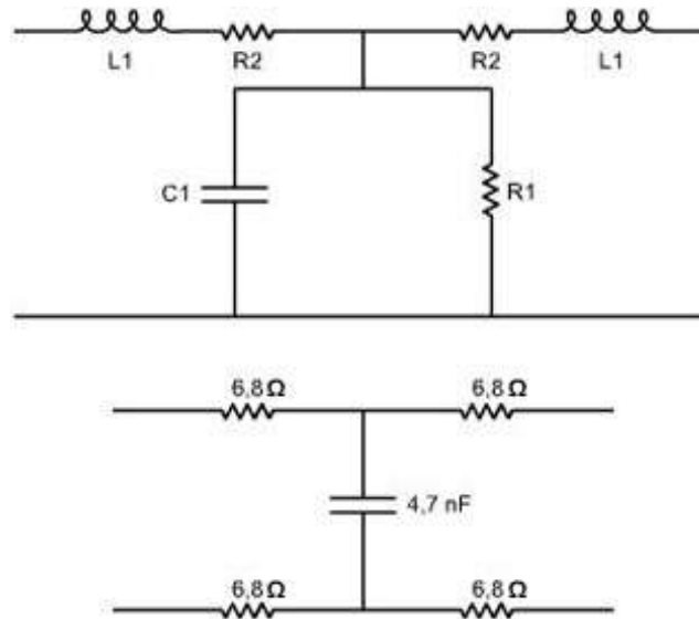
Figura 2.6 – Filtro passa-baixa representando a linha telefônica de 0,1 km
