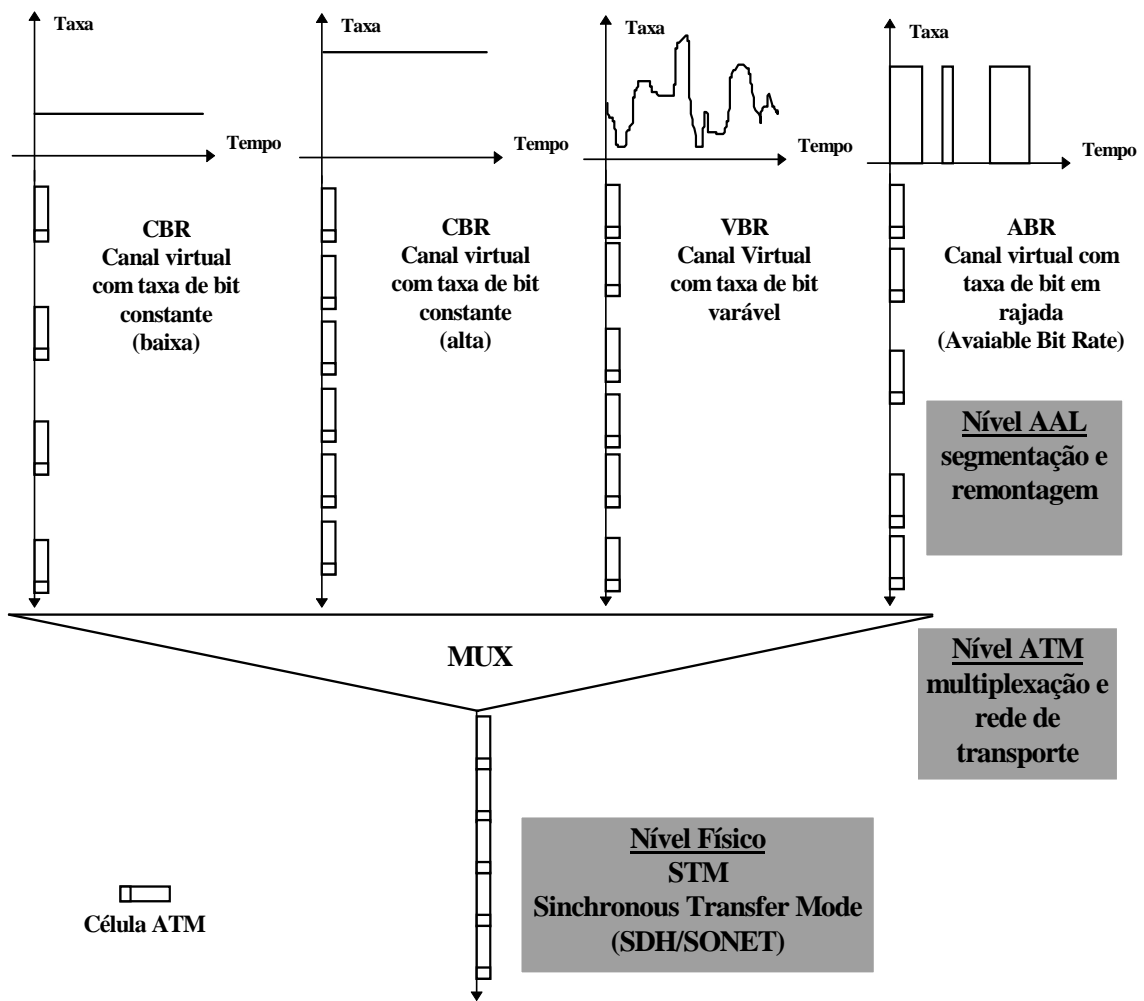
Figura 2.1 - O conceito básico de ATM
