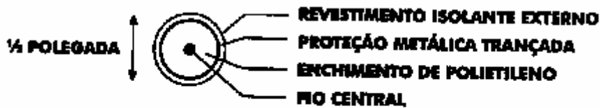
Figura 2.1 Um corte transversal no cabo coaxial usado na Ethernet original.
