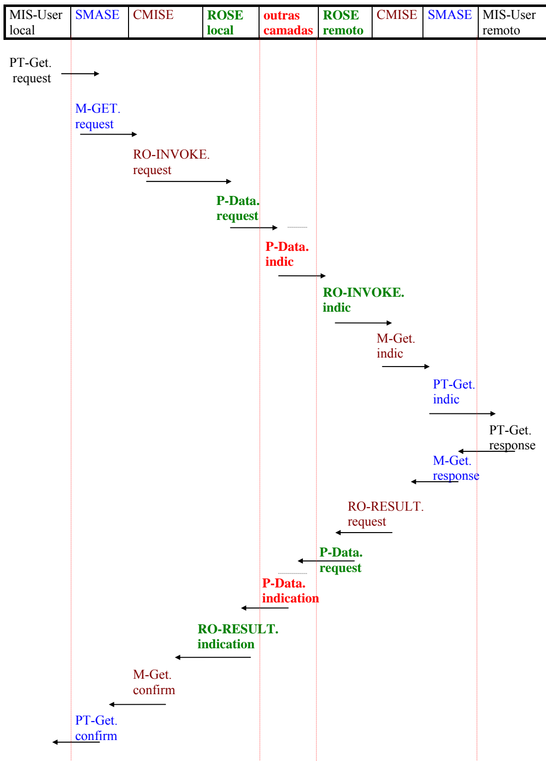
Figura 17.4 - Cenário de comunicação para a operação de leitura de valor de atributo
