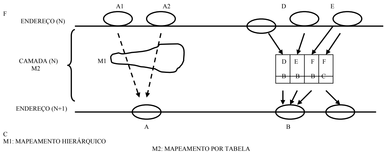
Figura 7.7: Tipos de mapeamento entre Endereços (N) e Endereços (N-1).
