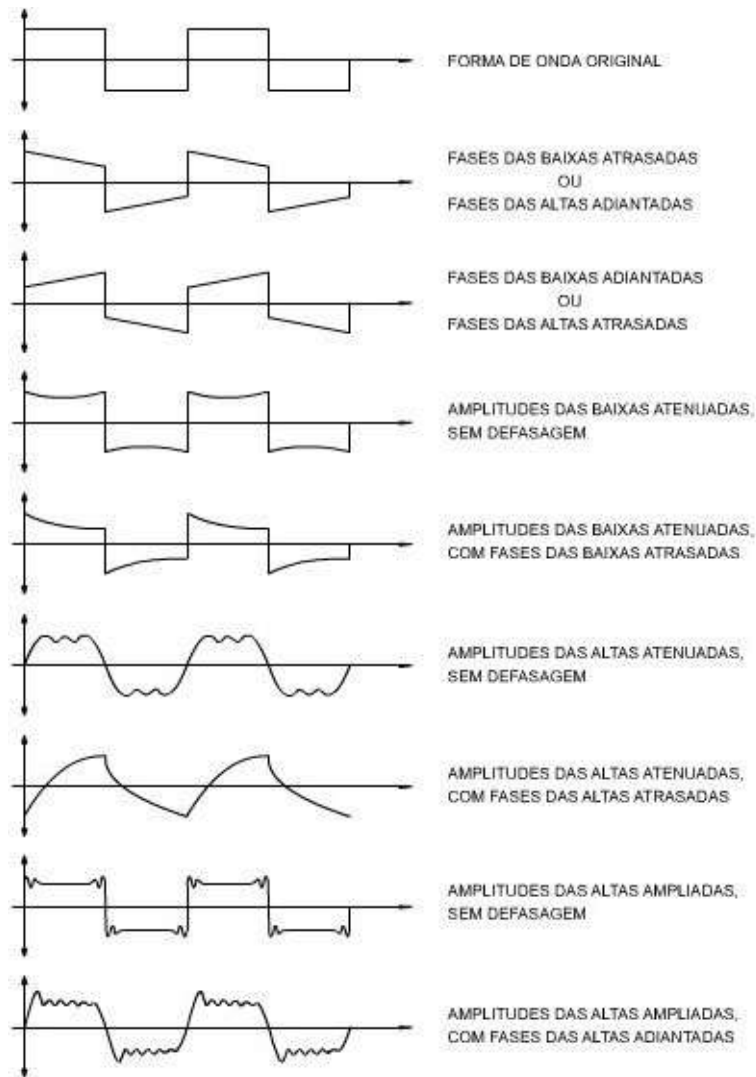
2.10 – Interpretação das distorções na onda quadrada
