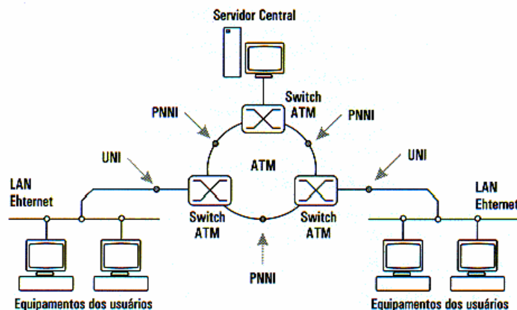
Figura X.5. Interfaces da tecnologia ATM.
