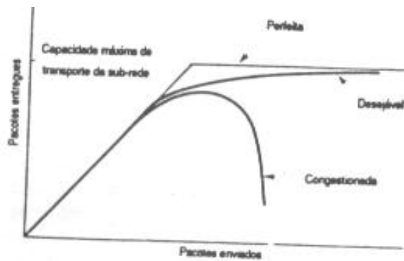
Figura 10-9 Quando é oferecido tráfego em demasia, vem o congestionamento, e o desempenho se degrada nitidamente.
