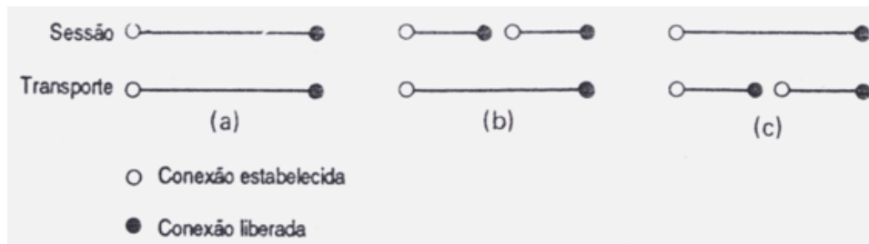
Figura 14.2. Três formas de mapear sessões sobre conexões de transporte
