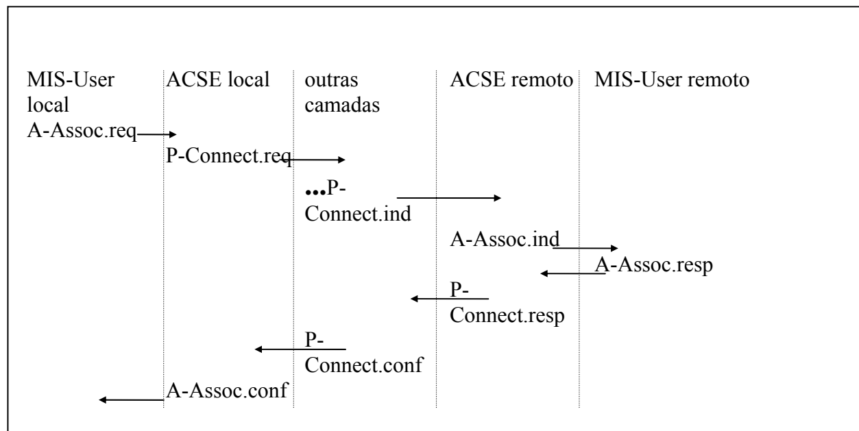
Figura 17.3- Fase de Associação entre dois MIS-Users
