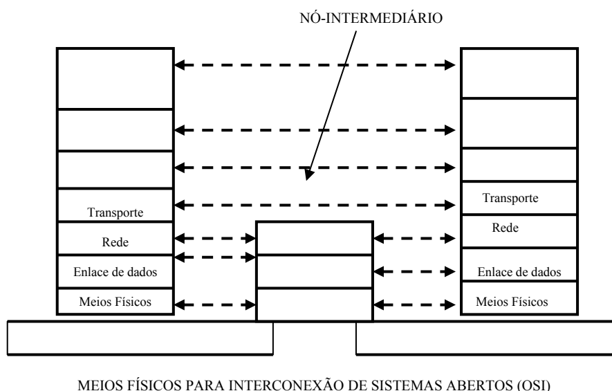
Figura 7.5: As setes camadas para a arquitetura OSI.
