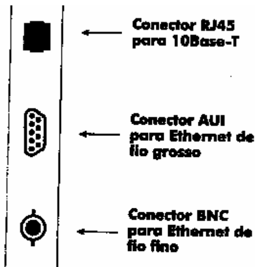
Figura 2.7 Um típico cartão adaptador da Ethernet com três conectores para os três esquemas de fiação da Ethernet. Apesar de o adaptador possuir três conectores, só um esquema de fiação pode ser utilizado por vez
