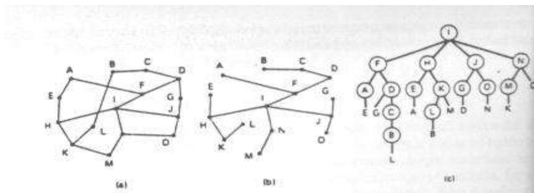
Figura 11-11 Progressão pelo caminho inverso
