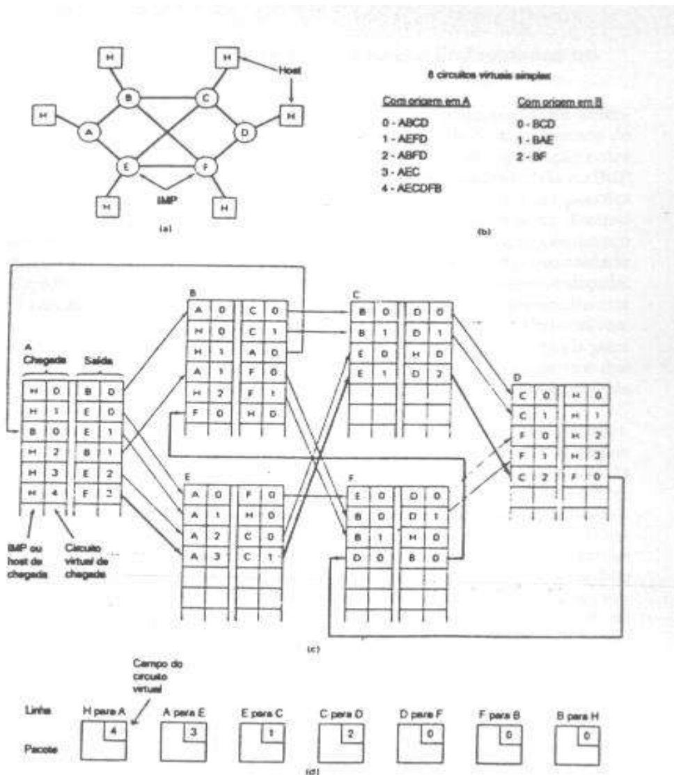
Figura 10-6 (a) Sub-rede de exemplo (b) Oito circuitos virtuais através da sub-rede (c) Tabelas do IMP para os circuitos virtuais em (b) (d) As mudanças no circuito virtual como uma progressão de pacote
