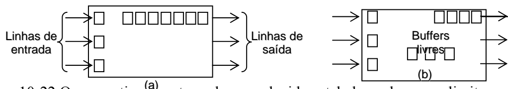
Figura 10-22 O congestionamento pode ser reduzido estabelecendo-se um limite superior para o número de buffers enfileirados em uma linha de saída
