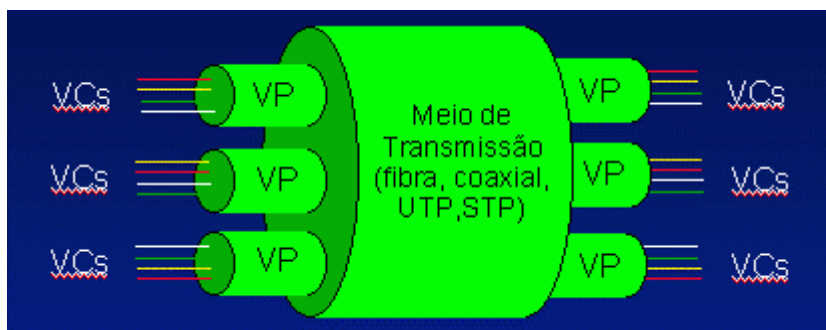
Fig. 2.8 Estrutura de Comutação ATM
