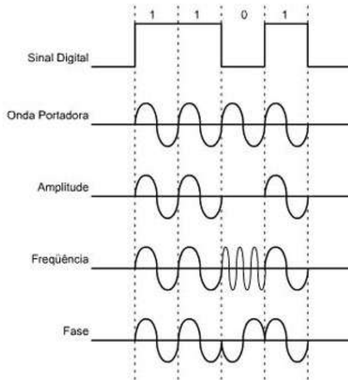
Figura 2.4 – Formas de Modulação
