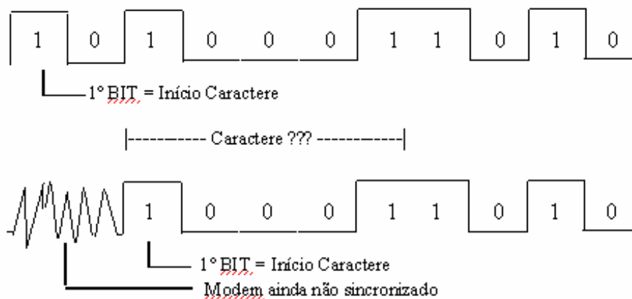
Figura - Sincronismo de Caracteres
